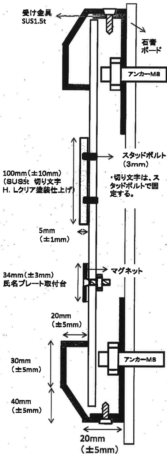
付図2一構造・材料・寸法(側面図)
